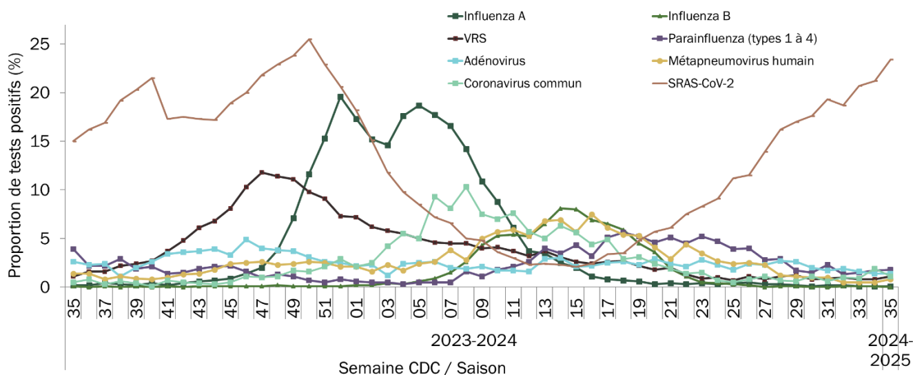
Graphique 5 : Pourcentage de tests positifs pour certains virus respiratoires, par semaine CDC, ensemble du Québec, saisons 2023-2024 & 2024-2025 (en cours)
